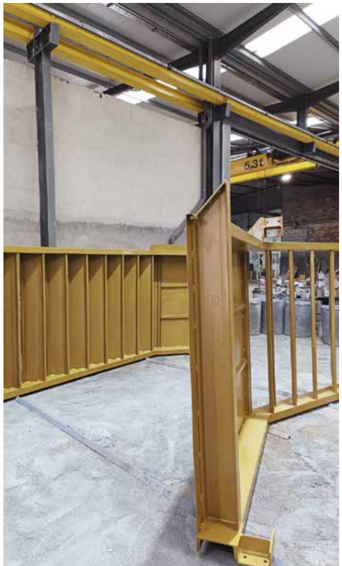
Obra: Estruturas metálicas // Localidade: Barcelos // Produtos: Primário Fosfato Zinco EP 15-410 + Esmalte Policril Metalizado RAL 1036 // Cliente: J. Mano & Cardante, Lda. // Comercial: Carlos Oliveira
