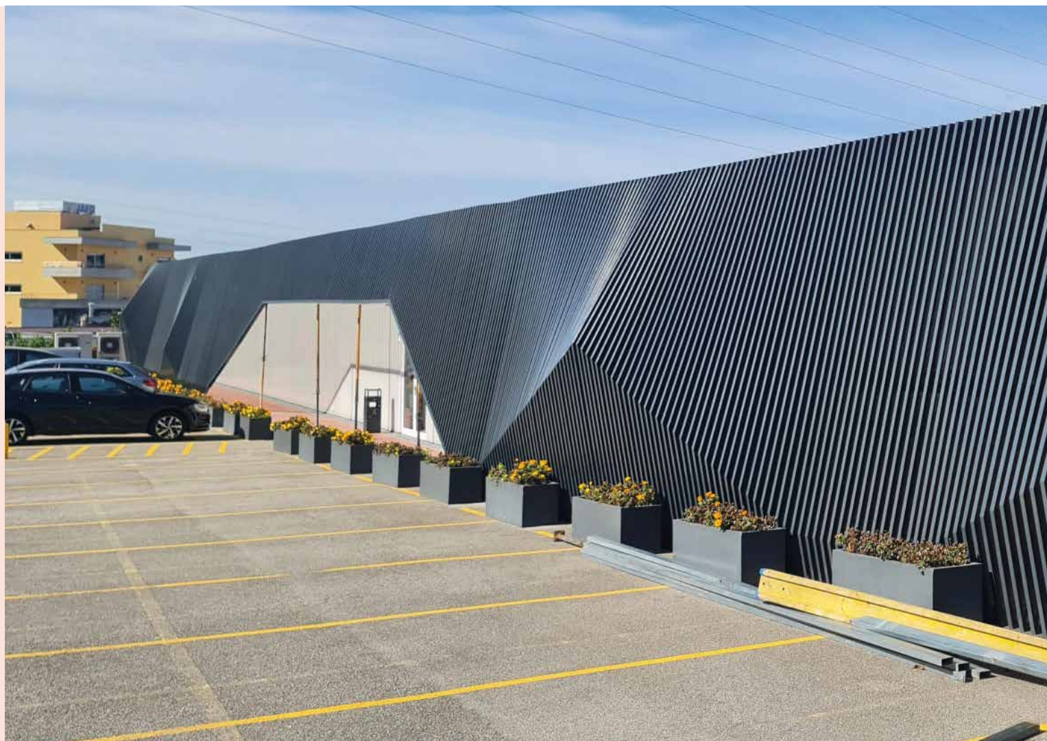
Obra: Biblioteca da Universidade CESPU // Localidade: Gandra - Paredes // Produtos: Esmalte Acrílico HB Gal RAL 7016 // Ciente: Serralharia Rui & Vieira, Lda.
